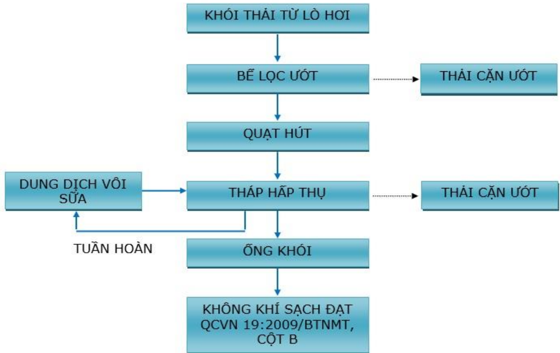
Hình 3. Sơ đồ hệ thống xử lý bụi, khí thải lò hơi
