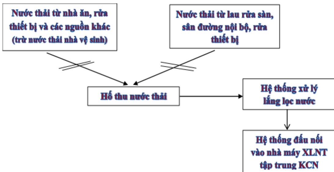
Hình 2. Sơ đồ quy trình thu gom, xử lý nước thải sinh hoạt khác và nước thải sản xuất
